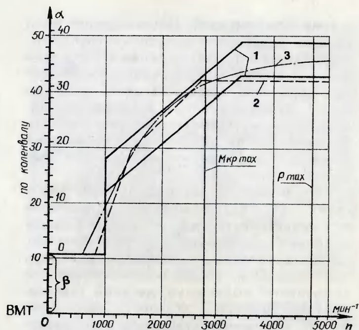
Графики зависимости угла опережения зажигания от частоты вращения коленвала распределителя Р107 для двигателя «Москвич—408»: 1 — приведенные в книгах «Ремонт автомобиля «Москвич» и «Электрооборудование автомобилей», упомянутых в тексте; 2 — характеристика, полученная автором; 3 — теоретическая характеристика, перестроенная в координаты для Р107.
