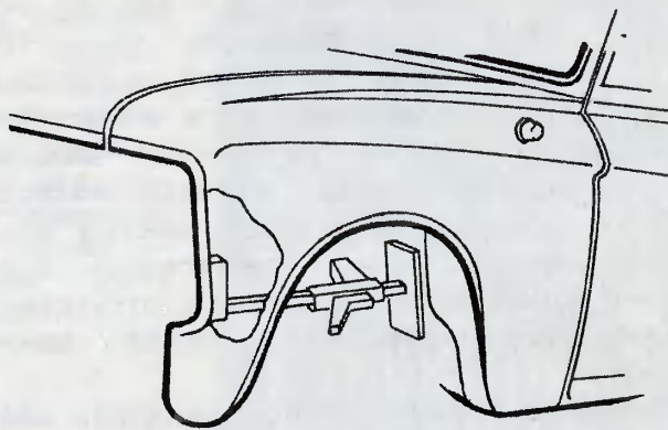
Так устанавливают для вытягивания крыла домкрат.
