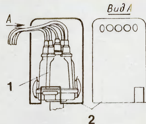
Защита распределителя (1) флаконом (2).
