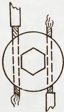
Соединение концов троса.
